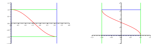
Graphes de cosinus cos| et arccosinus Arccos
