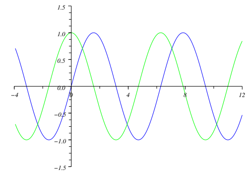
Graphes des fonctions sinus (en bleu) et cosinus (en vert)
