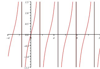
Graphes des fonctions tangente tg et arctangente Arctg
