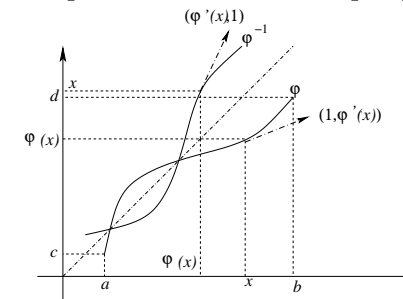
Graphe de la fonction réciproque
