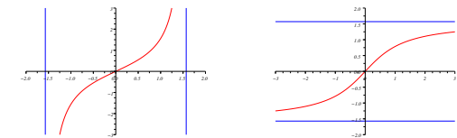
Graphes de tangente tg| et arctangente Arctg
