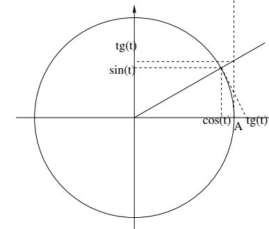
Le cercle trigonométrique
