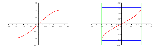
Graphes de sinus sin| et arcsinus Arcsin
