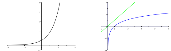
Graphes des fonctions Exponentielle et Logarithme
