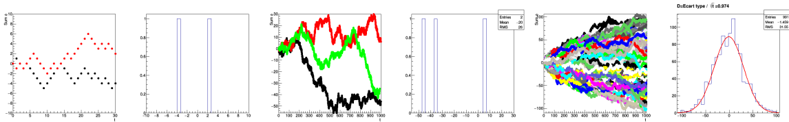
FIGURE 1.1 – Histogrammes pour Pile ou Face . A gauche représentation de S_t := \sum_{t'=1}^t x_{t'} où x_{t'} = \pm 1 sont aléatoires équadistribués. A droite, c'est l'histogramme de S_t à t = 30 avec N = 2 tirages, puis t = 1000 avec N = 3 puis N = 991 tirages. Dans ce dernier cas on observe que la distribution est bien ajustée par une Gaussienne avec un coefficient de diffusion \sigma = \sqrt{\frac{\text{Var}(S_t)}{t}} = 1 . Voir vidéo section 2.6 .
