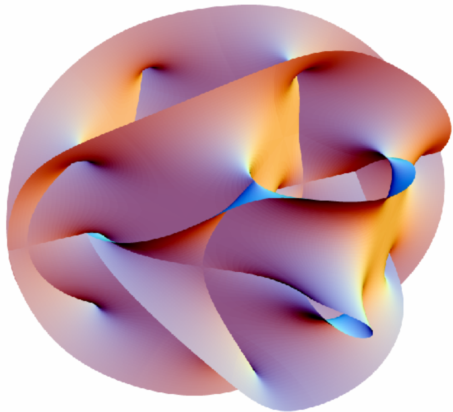
Structures métriques
