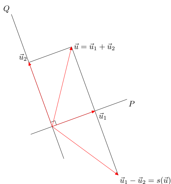
FIGURE 8. Symétrie orthogonale
