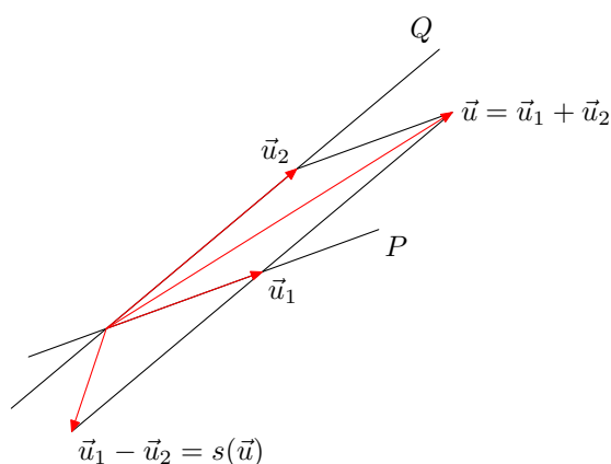
FIGURE 6. Symétrie par rapport à un sous-espace
