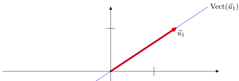
FIGURE 3. Sous-espace vectoriel engendré par un vecteur non nul
